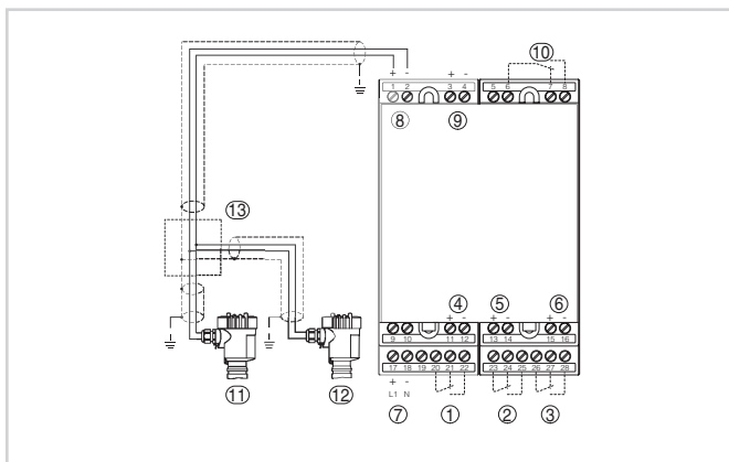
Подключение VEGAMET 625 и двухпроводных датчиков
